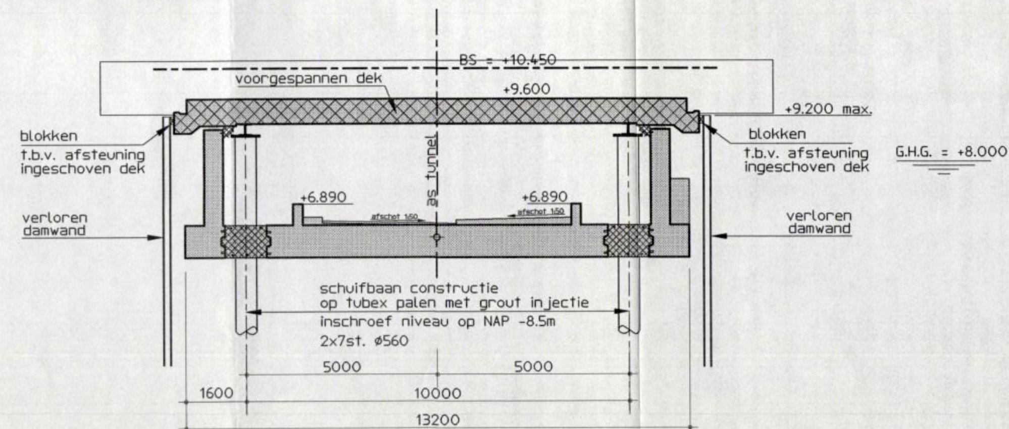
Dsn b 1:100
